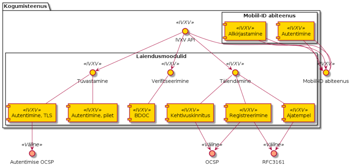
Joonis 2.3. Kogumisteenuse laiendusmoodulid ja välised teenused
