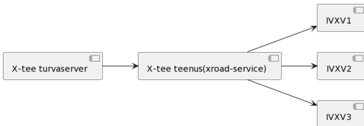
Joonis 1.1. X-tee teenus turvaserveri ja EHS-ide vahel
